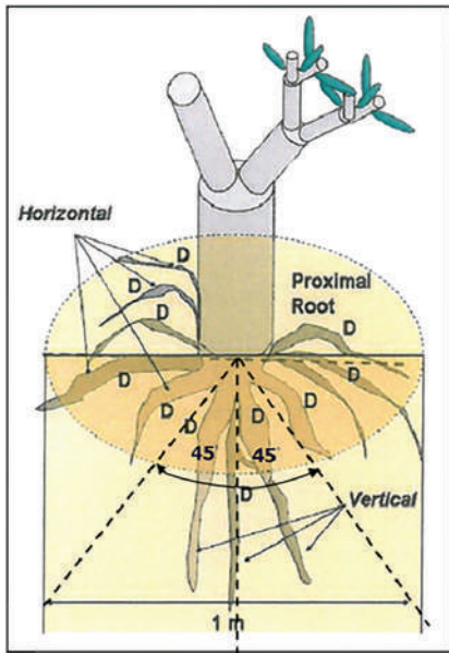
รูปที่ 4-23 การศึกษาระบบรากไม้ด้วยวิธีการคำนวณดัชนีความสามารถในการยึดดิน
