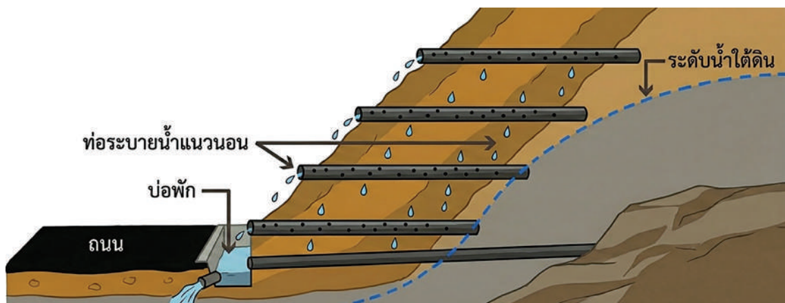
รูปที่ 2-24 ระบบระบายน้ำหลังลาด (subsurface drains) ที่มา : ดัดแปลงจาก Road Geohazard Risk Management Handbook 38
