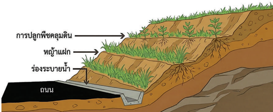
รูปที่ 2-22 การใช้วิธีชีววิศวกรรม (bioengineering) ที่มา : ดัดแปลงจาก Road Geohazard Risk Management Handbook 36
