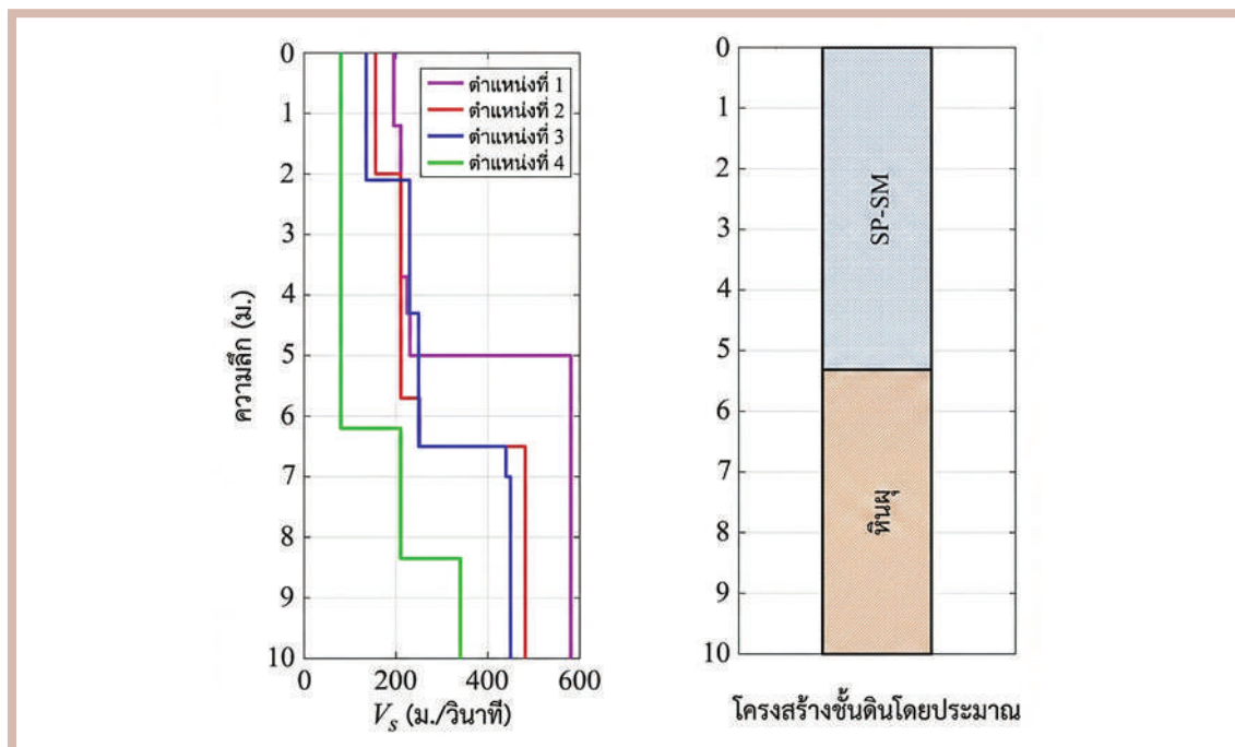
รูปที่ 2-10 ตัวอย่างการใช้ผลความเร็วคลื่นเฉือนเพื่อประมาณโครงสร้างชั้นดิน 22
