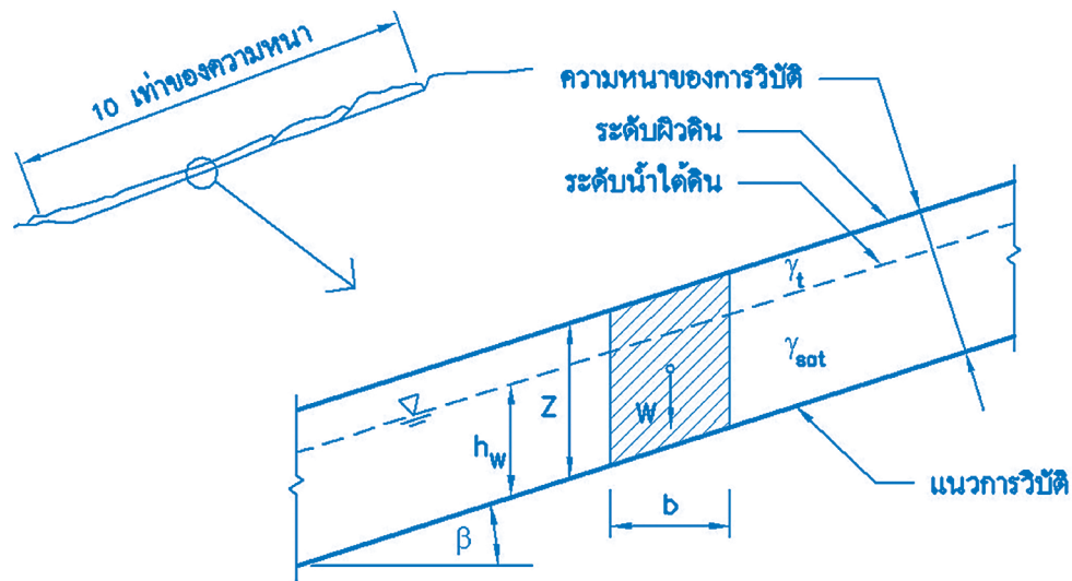
(ก) การเลื่อนไถลแบบระนาบ
