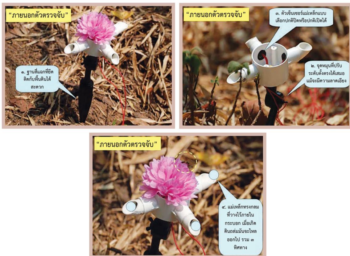
รูปที่ 4-27 ตัวตรวจจับการเคลื่อนตัวของน้ำและดิน (แบบที่ 1)
