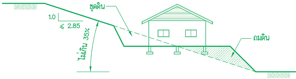
(ก) กรณีลาดเชิงเขาที่มีความชันไม่เกิน 1:2.85 (ร้อยละ 35)
