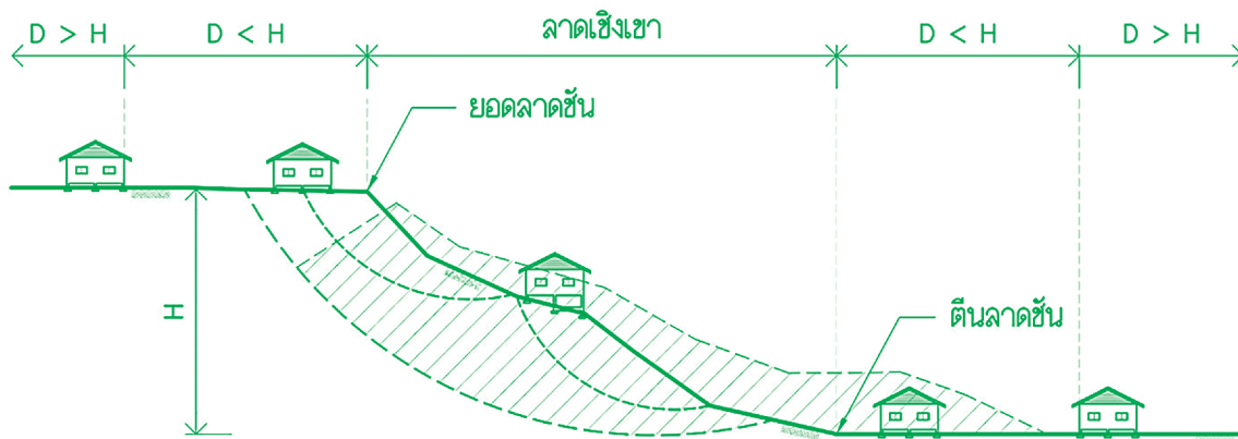
รูปที่ 2-32 ตำแหน่งของอาคารบริเวณพื้นที่ลาดเชิงเขา ที่มา : มาตรฐานกรมโยธาธิการและผังเมือง (2562) 46
