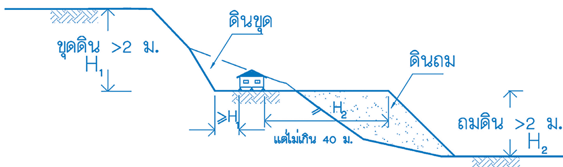
รูปที่ 2-37 ระยะเว้นเมื่อมีการถมดินและขุดดินบริเวณพื้นที่ลาดเชิงเขา
