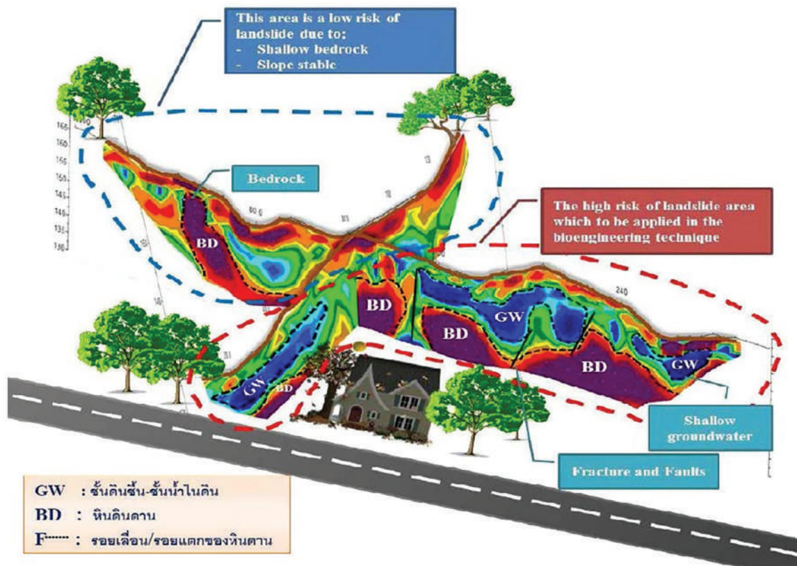
รูปที่ 4-7 สภาพทางธรณีวิทยาใต้ผิวดิน บริเวณที่มีปัจจัยเสี่ยงต่อการพังถล่ม (น้ำตกแม่พูล อำเภอลับแล จังหวัดอุตรดิตถ์)
