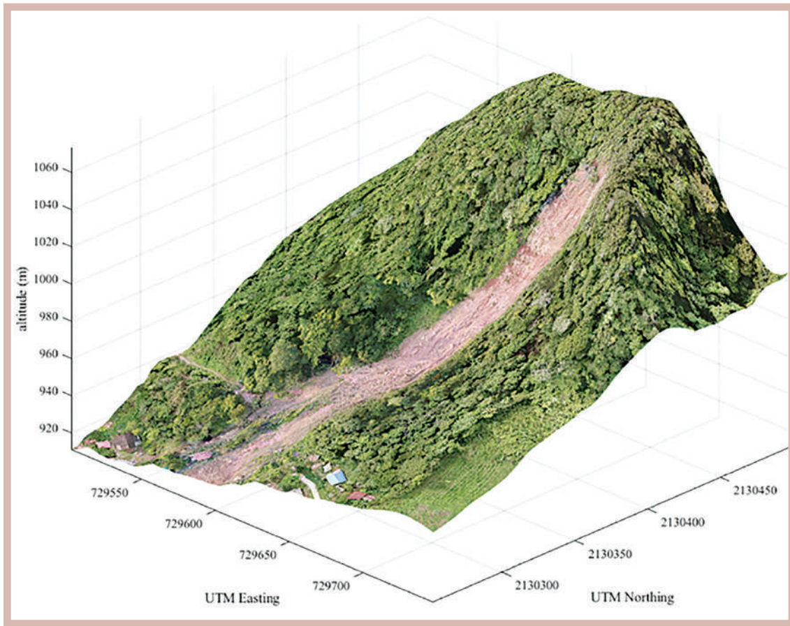
รูปที่ 2-7 ตัวอย่างแบบจำลอง DEM บริเวณตำแหน่งดินถล่มบ้านห้วยขา อำเภอบ่อเกลือ จังหวัดน่าน 22
