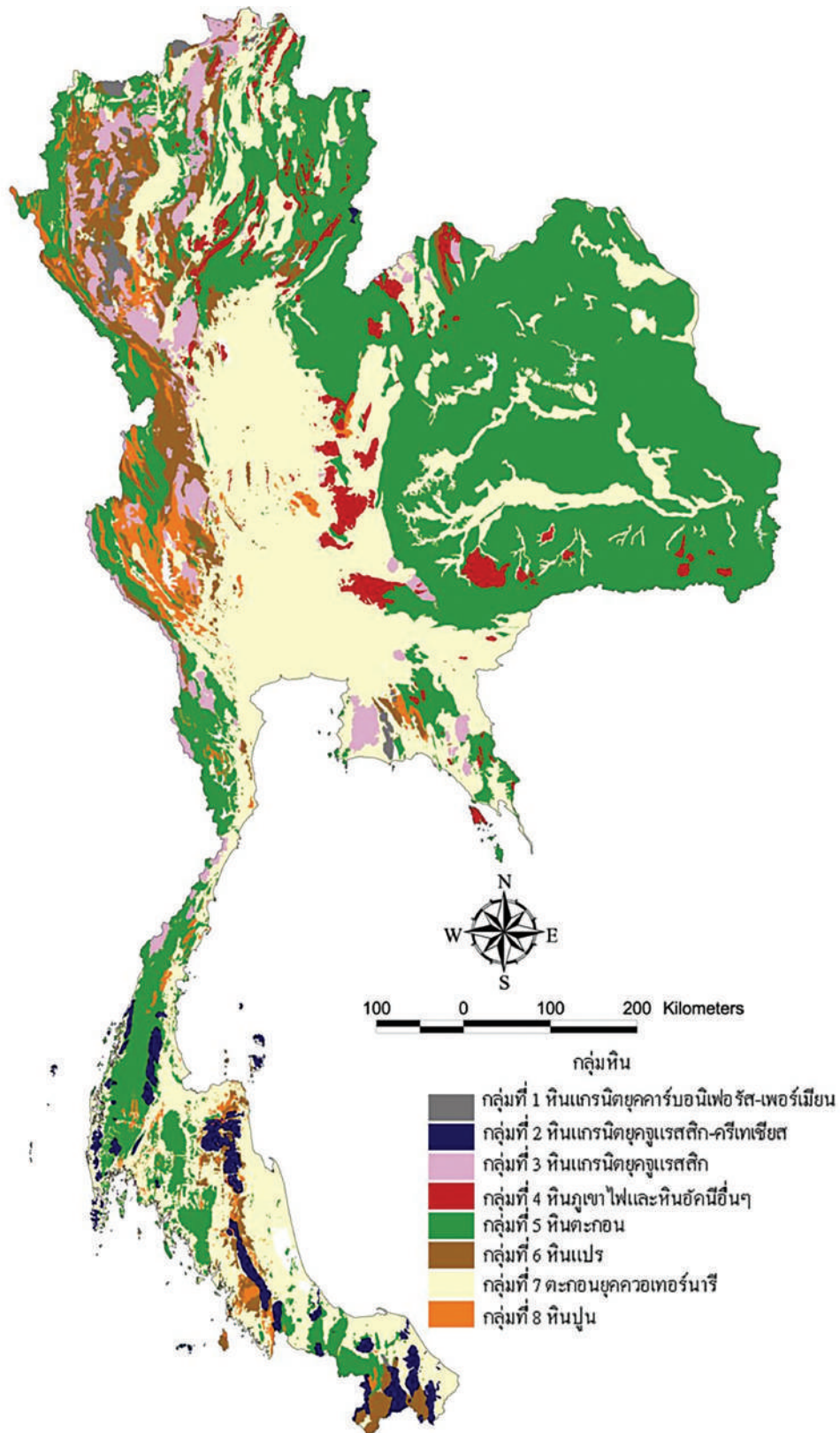
รูปที่ 2-2 การจำแนกทางธรณีวิทยาที่สำคัญทั้ง 8 กลุ่ม 17
