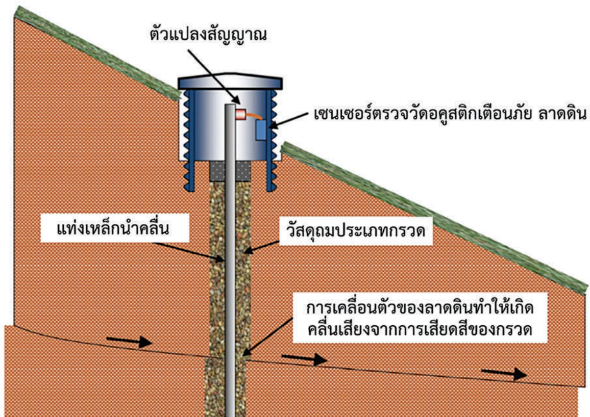
รูปที่ 3-19 อุปกรณ์เตือนภัยดินโคลนถล่ม โดยวิธีตรวจวัดคลื่นอคูสติก ที่มา : ดัดแปลงจาก Dixon และคณะ (2018) 74
