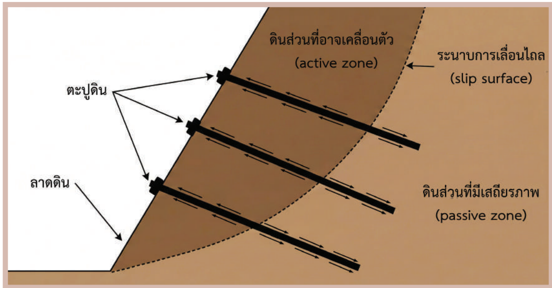
รูปที่ 3-14 กระบวนการเกิดแรงดึงในระบบตะปูดิน (soil nailing) ที่มา : ดัดแปลงจาก FHWA (2015)
