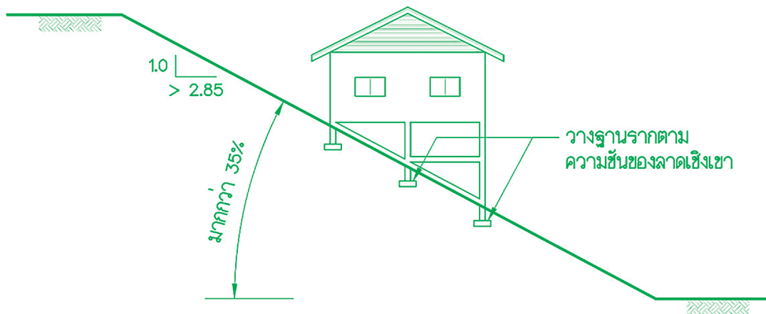
(ข) ลาดเชิงเขาที่มีความชันมากกว่า 1:2.85 (ร้อยละ 35)
