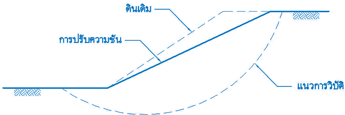
(ข) การปรับความชันของพื้นที่ลาดเอียง
