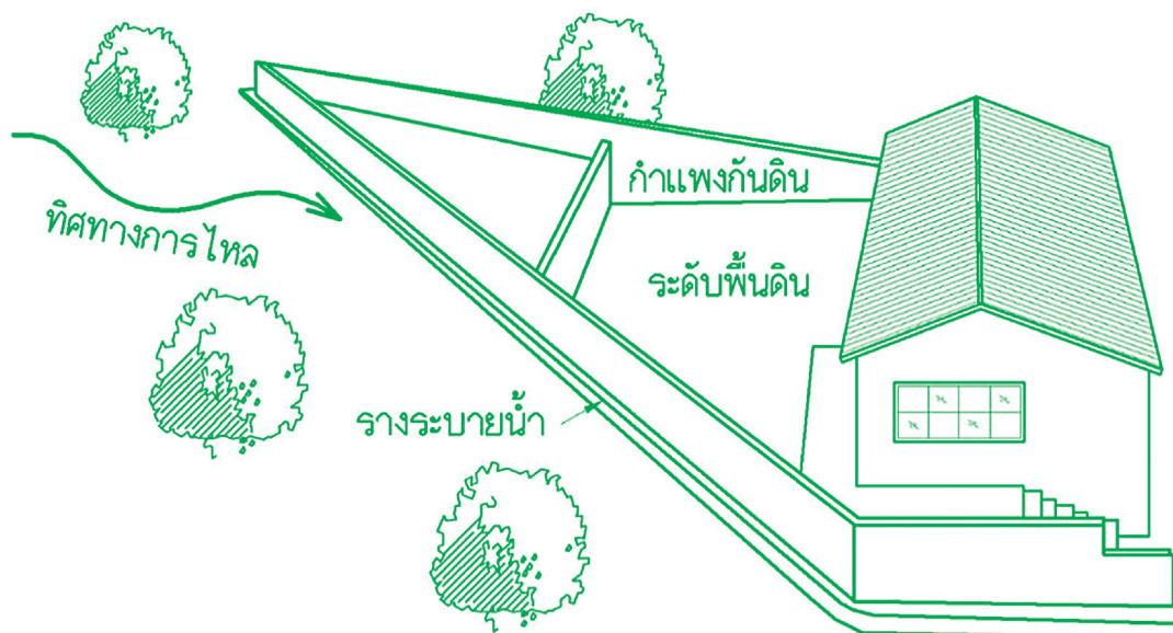
(ข) โครงสร้างเขียงทิศทางการไหลดินโคลนถล่ม
