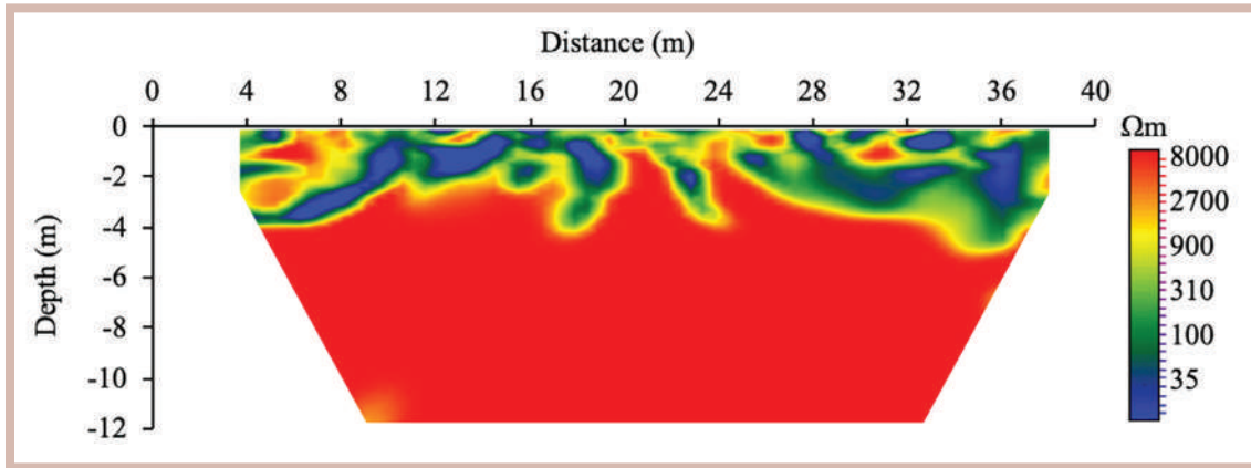
รูปที่ 2-9 ตัวอย่างผลวิเคราะห์ค่าความต้านทานทางไฟฟ้าของดิน 22
