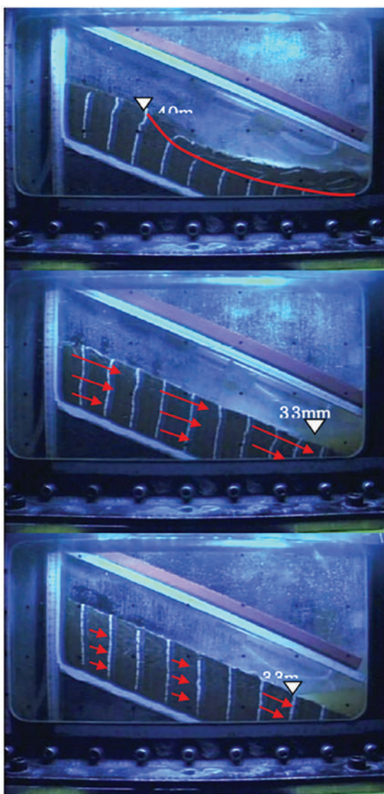
รูปที่ 4-17 ผลการจำลองพฤติกรรมการเสริมแรงของรากหญ้าแฝกบนลาดดินด้วยแบบจำลองหมุนเหวี่ยง
