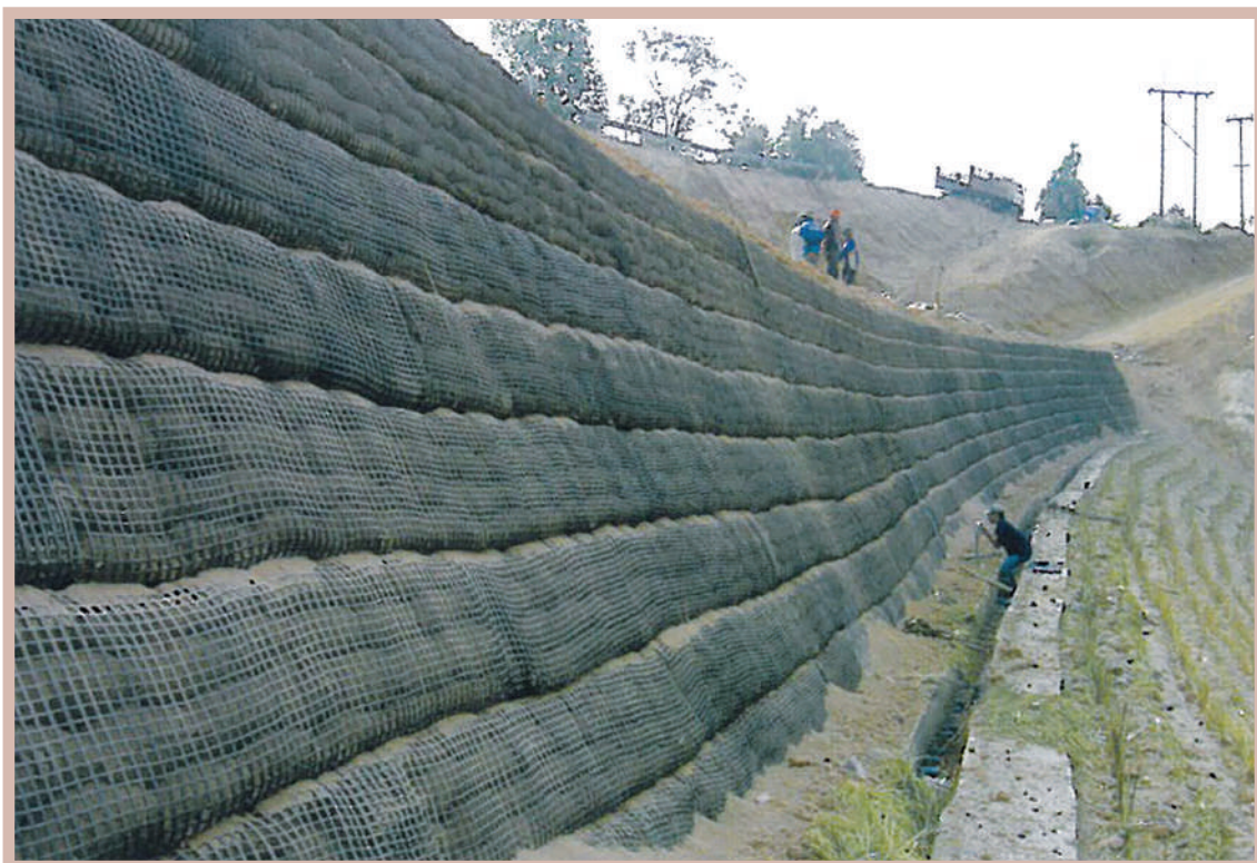
รูปที่ 3-15 ลาดดินเสริมแรงด้วยตาข่ายสังเคราะห์และปิดผิวหน้ากระสอบดิน (reinforced soil slope with geogrid reinforcement and soil bag facing)
