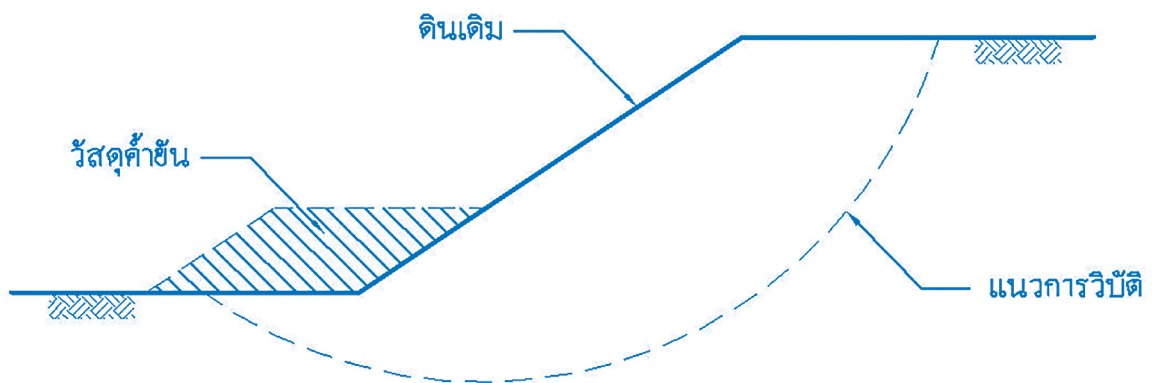
รูปที่ 2-35 การใช้น้ำหนักยันบริเวณฐานพื้นที่ลาดเอียง ที่มา : มาตรฐานกรมโยธาธิการและผังเมือง (2562) 49
