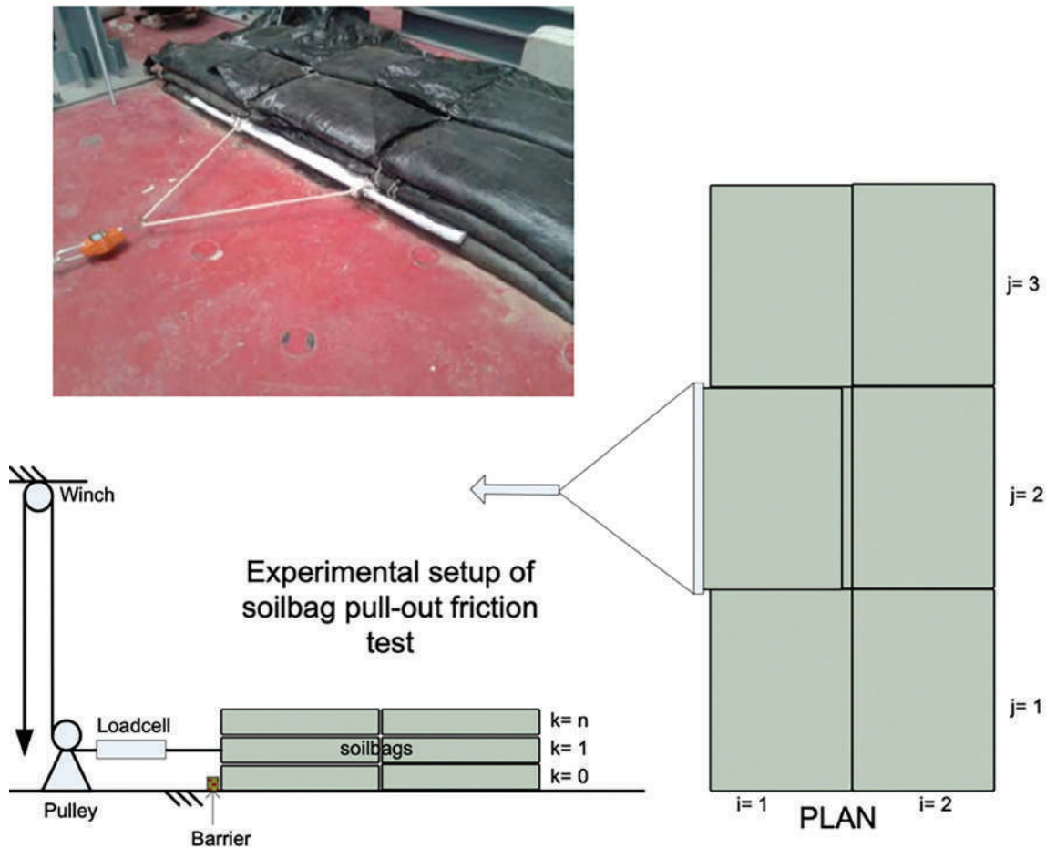
รูปที่ 4-20 การทดสอบแรงเสียดทานระหว่างกระสอบมีปีก
