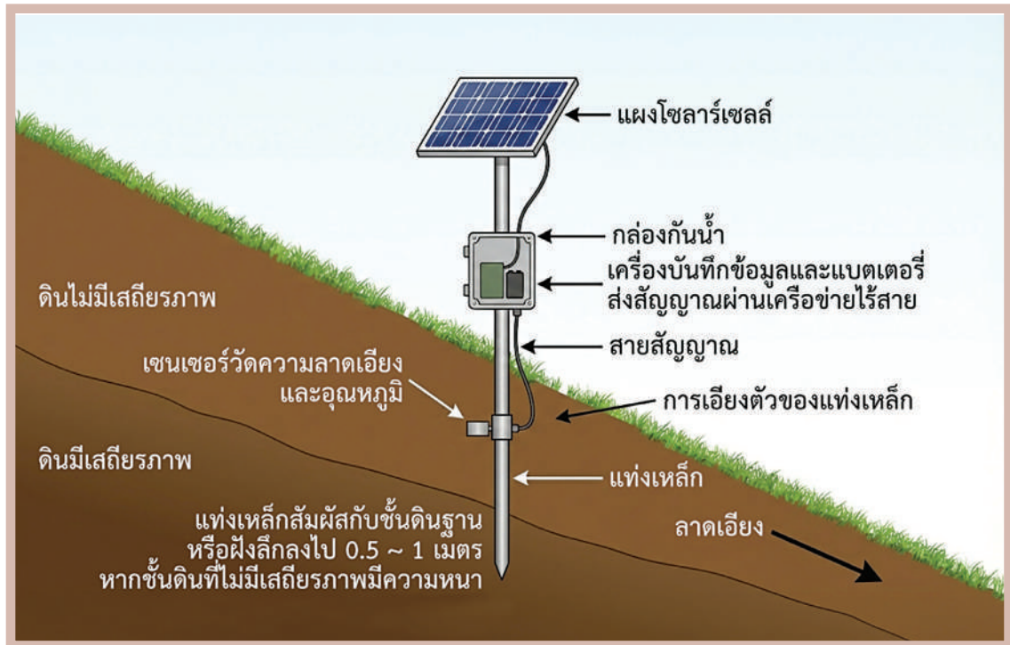
รูปที่ 3-18 การติดตั้งเครื่องมือวัดความลาดเอียงที่ผิวดิน (surface tilt meter) ที่มา : ดัดแปลงจาก Uchimura และคณะ (2013) 73
