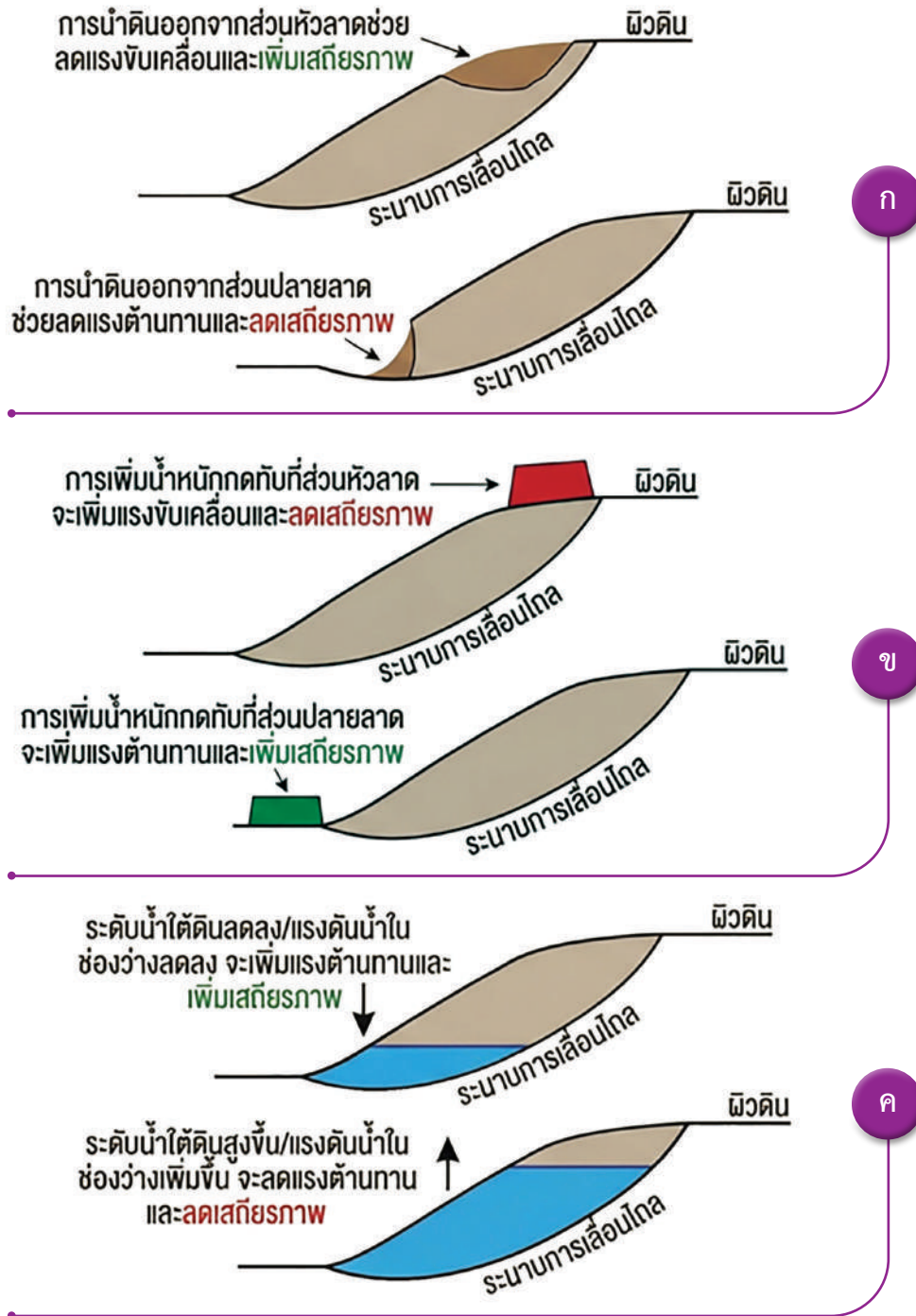
รูปที่ 3-8 การเพิ่มขึ้นหรือลดลงของเสถียรภาพลาดดิน (ก) ผลของการขุดดินที่ส่วนหัวและส่วนปลายของลาดดิน (ข) ผลของการเพิ่มน้ำหนักกดทับที่ส่วนหัวหรือส่วนปลายของลาดดิน (ค) ผลของการเปลี่ยนแปลงของระดับน้ำต่อเสถียรภาพของลาดดิน ที่มา : ดัดแปลงจาก Rex Baum, U.S. Geological Survey 57
