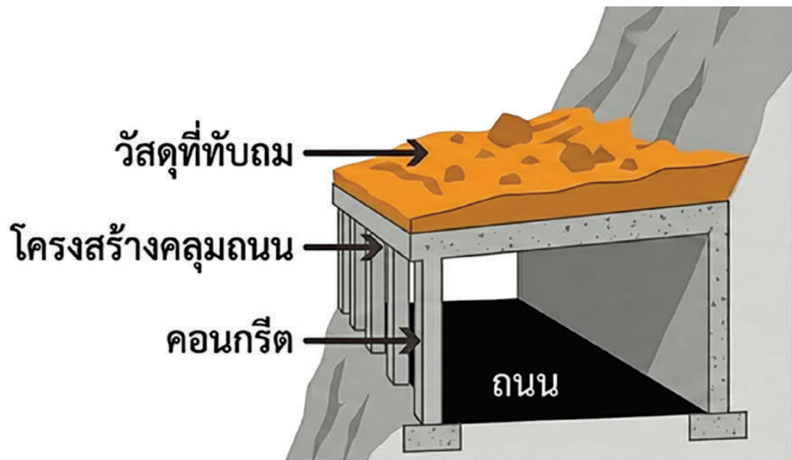
รูปที่ 2-20 โครงสร้างคลุมถนน (shelters) ที่มา : ดัดแปลงจาก Road Geohazard Risk Management Handbook 34
